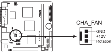
AT3GC-I fan connectors
