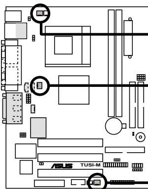
TUSI-M 12-Volt Cooling Fan Power
